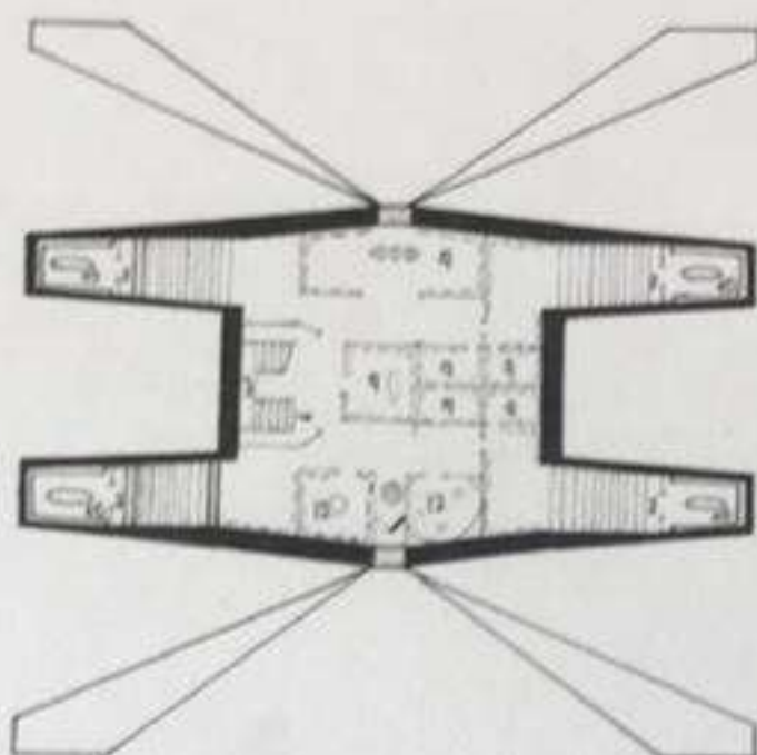
ПЛАН-2
